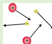
電離気体 (プラズマ)
